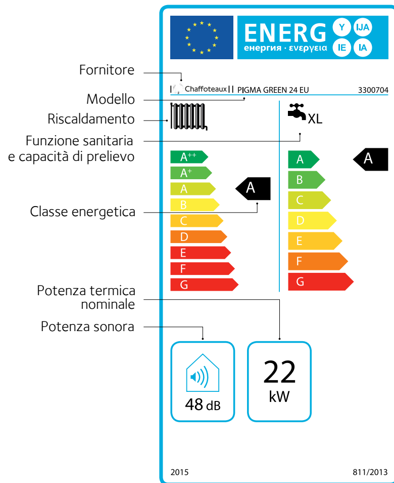
Etichetta energetica di una caldaia mista
